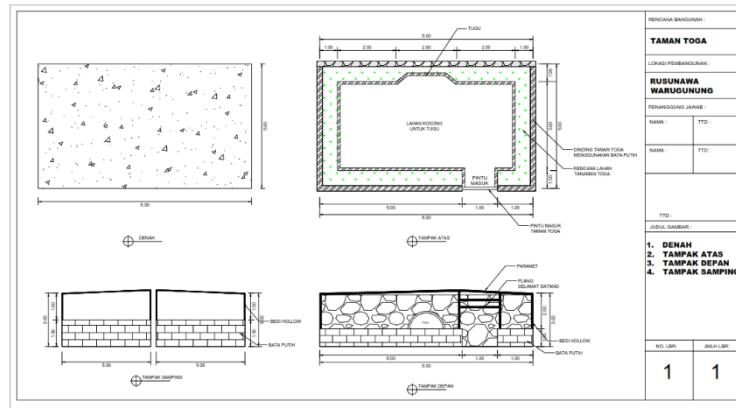
Gambar 4. Denah dan Desain Pembangunan Taman Toga
